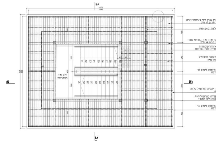
תכנית מפלס עליון קנ"מ 1:50
