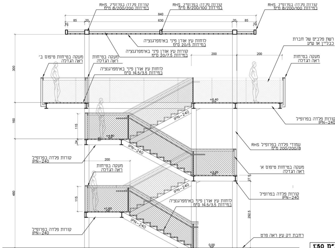
חתך א-א קנ"מ 1:50
